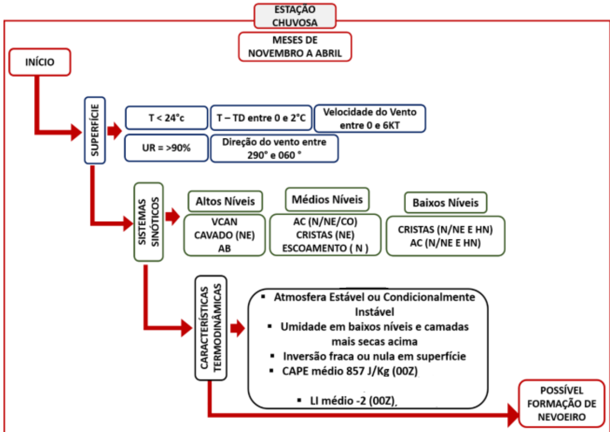
Figura 39: Método Operacional de previsão de Nevoeiro- Manaus/Estação Chuvosa. T – Temperatura do ar; TD – Temperatura do ponto de orvalho; UR-umidade relativa; VCAN – Vórtice Ciclônico de Altos Níveis; AB- Alta da Bolívia; AC- Anticiclone; N- Norte; NE- Nordeste; CO- Centro Oeste; CAPE- Energia Potencial de Convectiva Disponível; LI- Índice de Levantamento.
