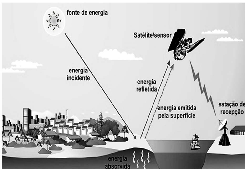
Figura 1 - Esquema do Sensoriamento Remoto.
