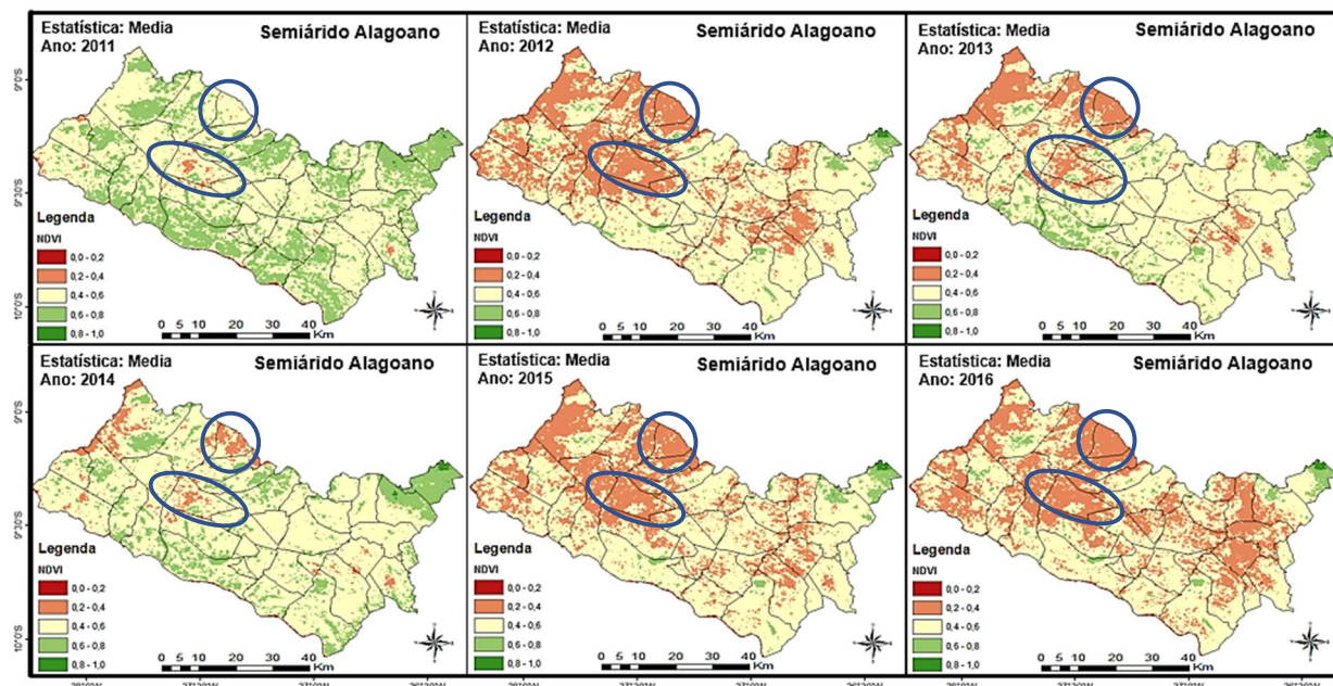
Figura 27 - Distribuição espaço-temporal da média interanual do IVDN do período de 2011 a 2016.
