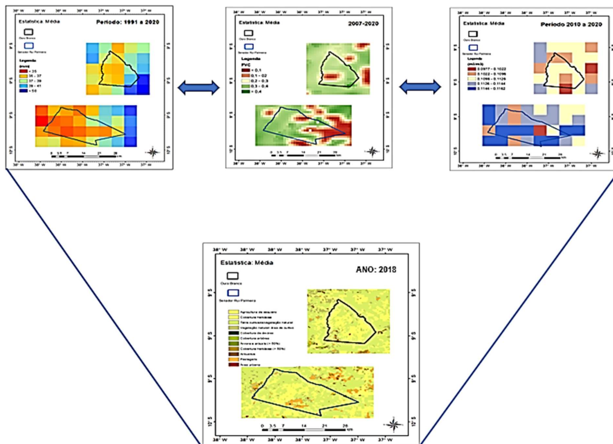
Figura 21 - Relação do FVC com precipitação e umidade do solo, comparando com as características do uso e cobertura do solo.
