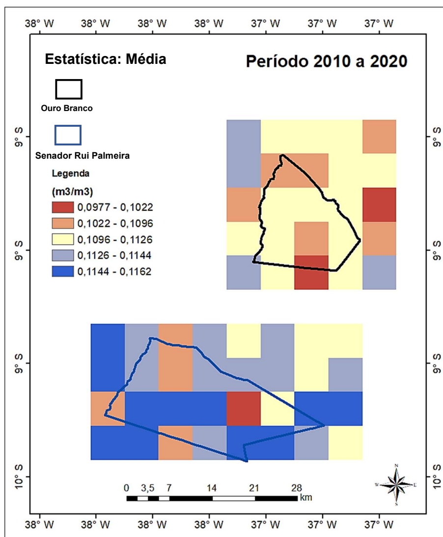
Figura 20 - Média interanual da umidade do solo, dos municípios Ouro Branco-AL e Senador Rui Palmeiras-AL (2010 a 2020).
