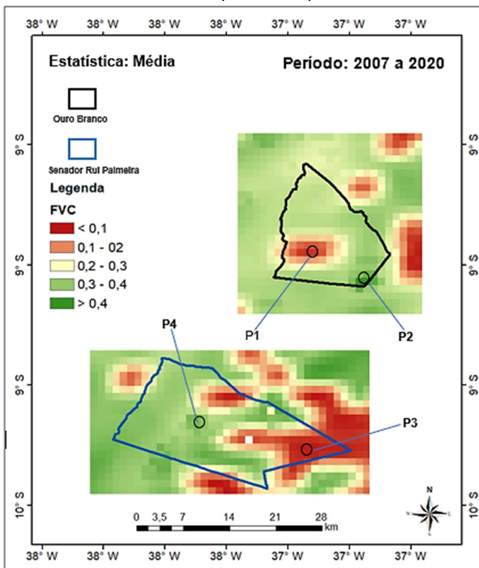
Figura 17 - Média interanual do FVC, dos municípios Ouro Branco-AL e Senador Rui Palmeiras-AL (2007 a 2020).
