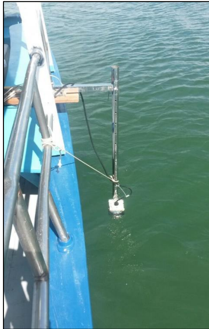
Figura 26: ADCP utilizado para medição da velocidade e direção da corrente.
