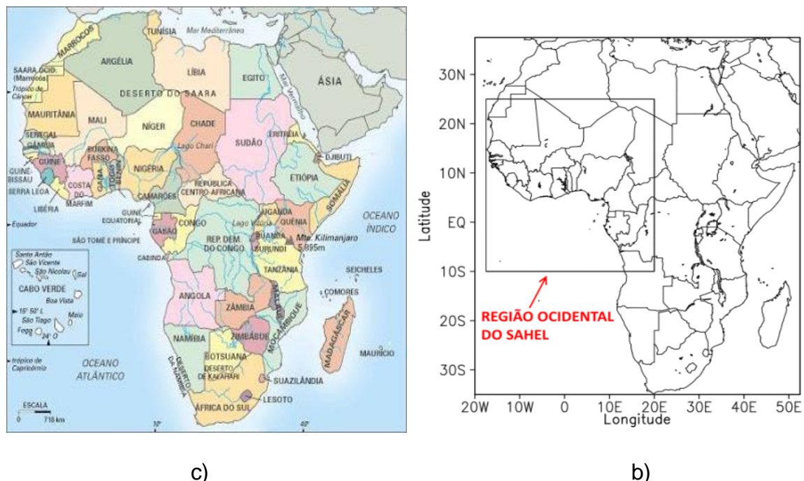
Figura 10 - Localização da área de estudo a) Continente Africano. b) Região do Ocidental Oeste do Sahel.
