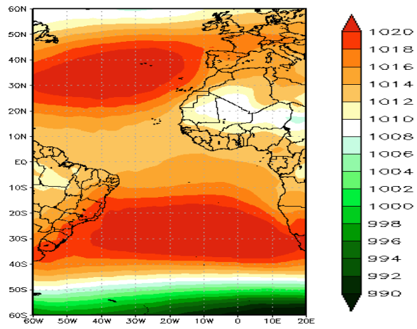
Figura 15 - Posição média b) deslocamento latitudinal e c) deslocamento longitudinal das altas subtropicais para a fase quente da ODP 1976-1998.
