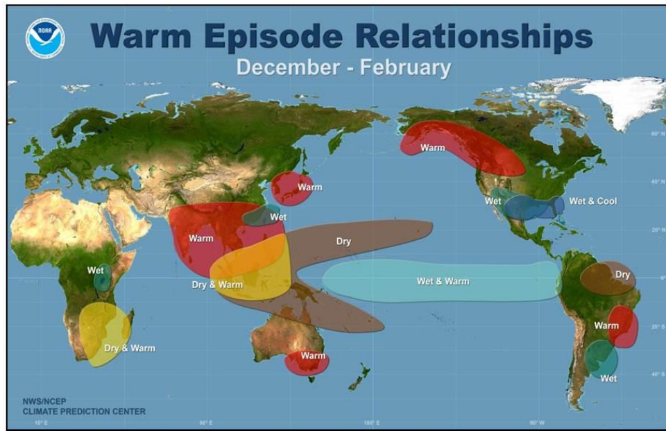
Figura 8 - Impacto do fenômeno El Niño em diversas partes do globo para a) verão e b) inverno.
