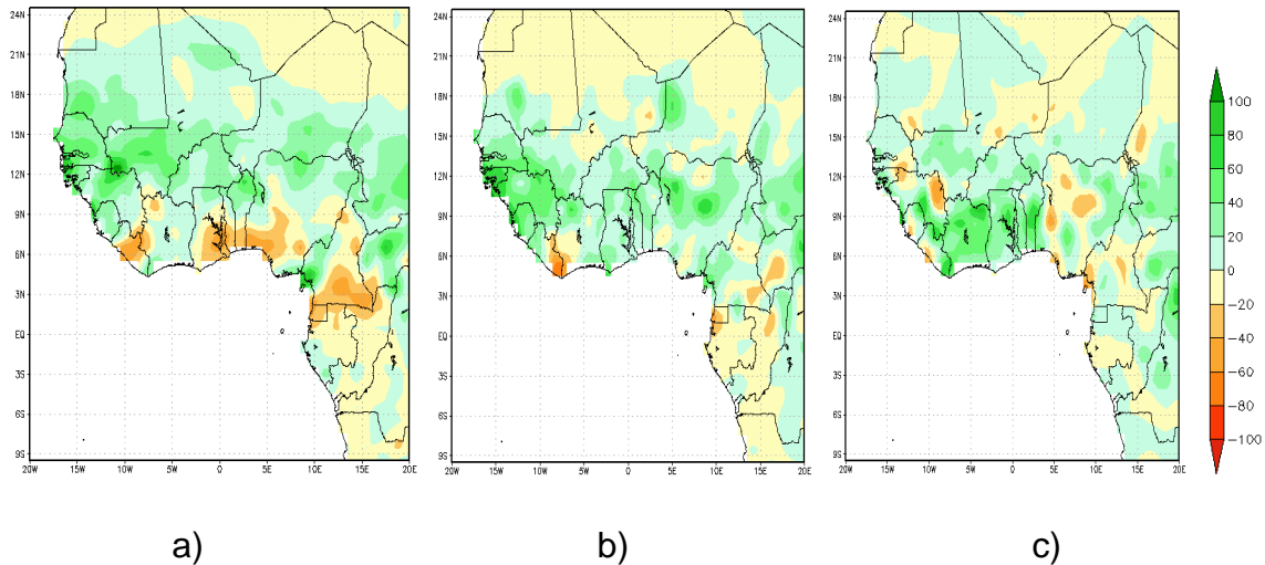
Figura 36 - Desvios de precipitação a)1954-1955 b)1975-1976 c) 1988-1989 d) 1997-1998 de julho-setembro com relação ao período 1948-2014, associado às La niñas de 1955, 1975, e 1989 respectivamente.
