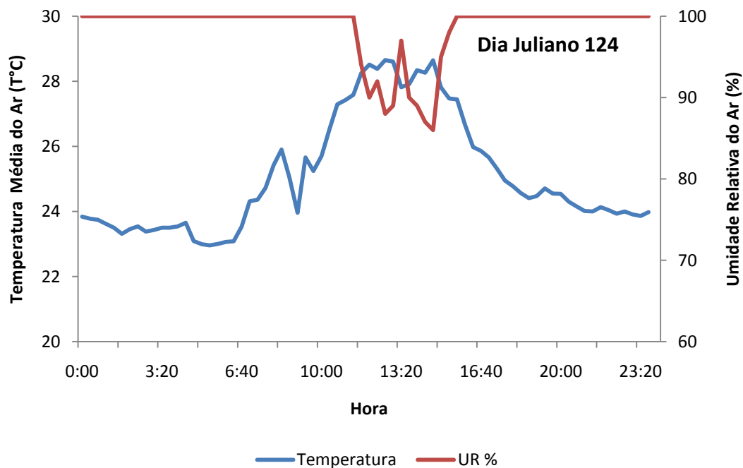
Figura 22 – Elementos do clima observados no dia 124.
