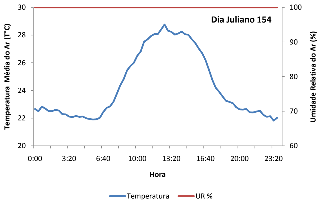
Figura 18 – Elementos do clima observados no dia 154.
