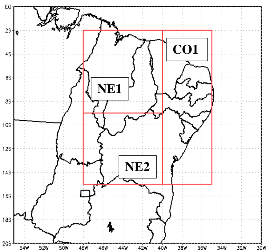
Figura 6 - Subdivisões das áreas para avaliação objetiva. NE1 (Maranhã, Piauí e parte do Ceara e Pernambuco), NE2 (Grande parte da Bahia, uma pequena porção do Piauí e uma parte do
