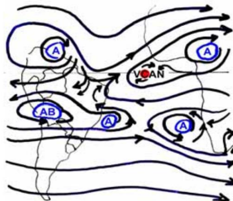
Figura 9 - Processo de formação do VCAN (Africana II).
