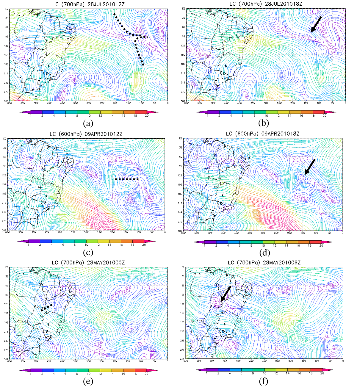
Figura 21 – Campos compostos de escoamento e magnitude do vento ( m s^{-1} ) em 700, 600 e 500 hPa mostrando exemplos dos processos de formação do Tipo III: Tipo IIIa (a, b), Tipo IIIb (c, d), Tipo IIIc (e, f) e Tipo III d (g, h). Evento do dia 28/07/2010 às 12 UTC (a) e 18 UTC (b). Evento do dia 09/04/2010 às 12 UTC (c) e 18 UTC (d). Evento do dia 28/05/2010 às 00 UTC (e) e 06 UTC (f). Evento do dia 02/05/2010 às 06 UTC (g) e 12 UTC (h). Linha tracejada: encontro das correntes e cavado. Setas: VCMN.
