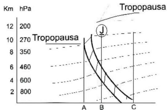
Figura 4 - Seção vertical, mostrando a zona de forte baroclinia na troposfera (entre A e C); zona frontal e corrente de jato (J), situada sobre a vertical B.
