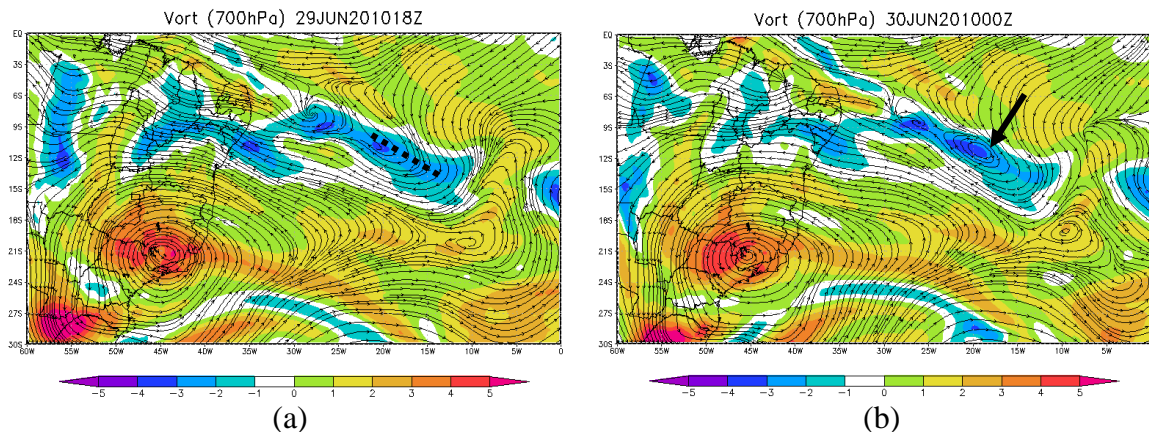
Figura 22 – Exemplos dos campos meteorológicos para os processos de formação do Tipo Ia: vorticidade ( \times 10^{-5} \text{ s}^{-1} ) (a, b), divergência ( \times 10^{-5} \text{ s}^{-1} ) (c, d), velocidade vertical ( \text{Pa s}^{-1} ) (e, f), e escoamento em 700 hPa para o dia 29/06 às 18 UTC e 30/06/2010 às 00 UTC. Coluna esquerda: pré- formação; coluna direita: VCMN formado. Linha tracejada: cavado. Seta: VCMN.
