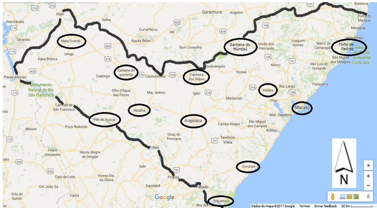
Figura 15 – Mapa do estado de Alagoas com as localizações das estações de superfície.
