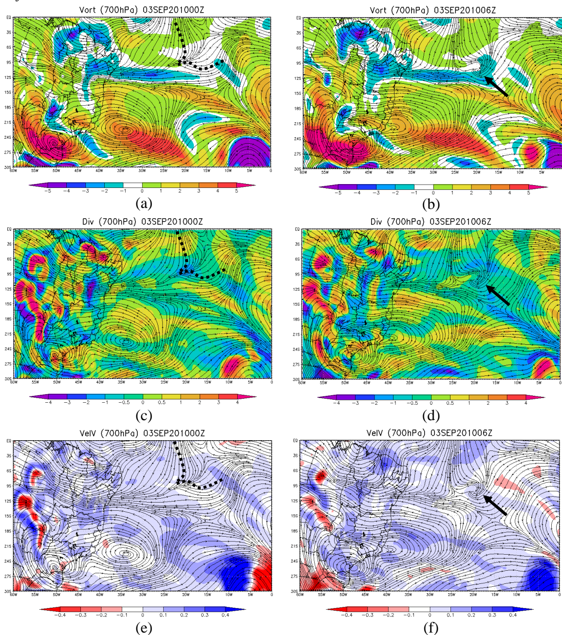
Figura 24 – Exemplos dos campos meteorológicos para os processos de formação do Tipo IIIa: vorticidade ( \times 10^{-5} \text{ s}^{-1} ) (a, b), divergência ( \times 10^{-5} \text{ s}^{-1} ) (c, d), velocidade vertical ( \text{Pa s}^{-1} ) (e, f), e escoamento em 700 hPa para o dia 03/09/2010 às 00 UTC e 06 UTC. Coluna esquerda: pré-formação; coluna direita: VCMN formado. Linha tracejada: encontro das correntes. Seta: VCMN.
