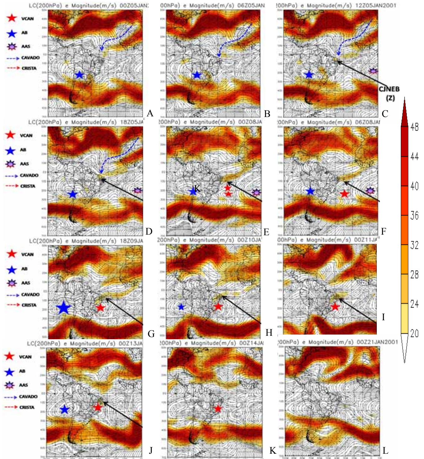
FIGURA 33 Linhas de corrente em 200 hPa e magnitude do vento ( m.s^{-1} ) em dias alternados no mês de janeiro de 2001.
